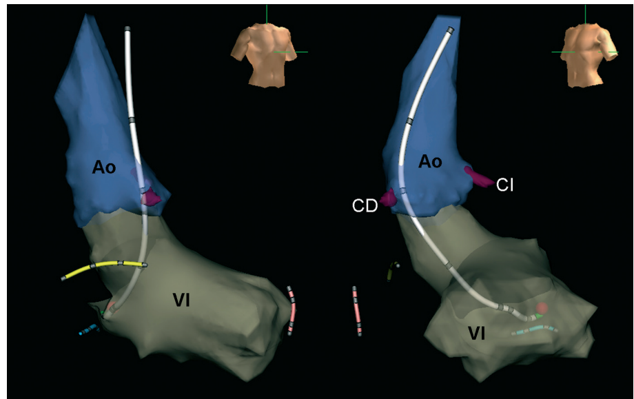
Fig. 2. Ablación de una vía accesoria auriculoventricular izquierda guiada mediante el sistema de navegación no fluoroscópica Ensight-NavX y sin utilización de un sistema de fluoroscopia. Se representan en visión oblicua anterior derecha (panel izquierdo) e izquierda (panel derecho) la reconstrucción anatómica virtual del ventrículo izquierdo (VI), la aorta (Ao), la coronaria izquierda (CI) y la coronaria derecha (CD), junto con un catéter de ablación de ocho polos de diseño propio (Therapy plus®, Irvine), situado en el punto de ablación eficaz (esfera roja), y tres catéteres diagnósticos situados en la región hisiana (amarillo), el seno coronario (azul) y el ápex del ventrículo derecho (rosa).
