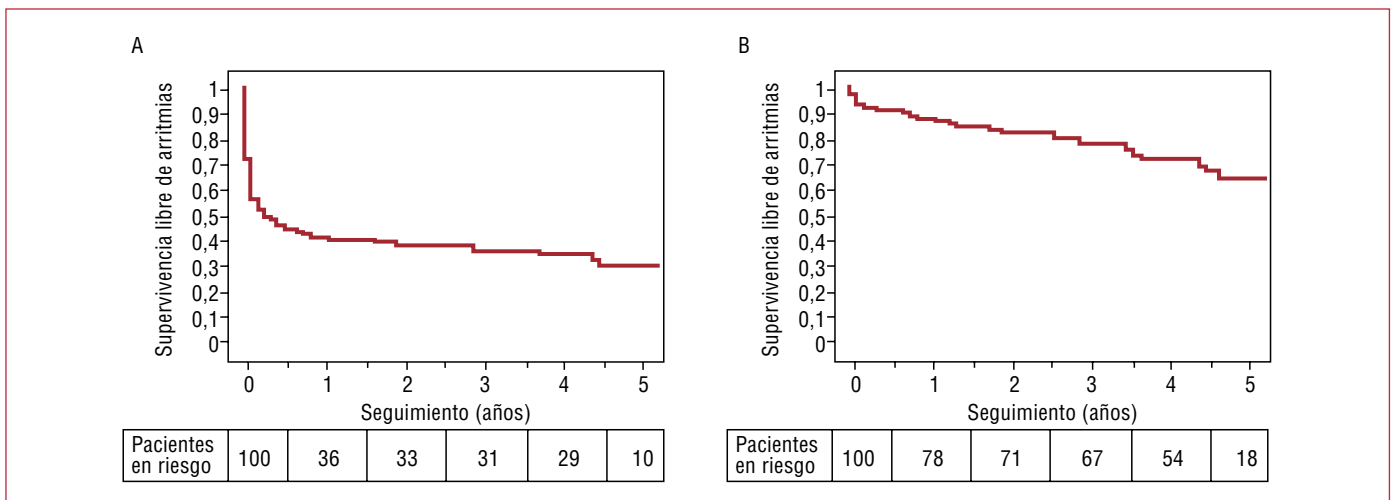
Figura 2. Éxito del procedimiento de ablación de la fibrilación auricular. Curvas de Kaplan-Meier de supervivencia sin arritmias tras un único procedimiento de ablación con catéter (A) y tras el último (múltiples) procedimiento (B). Adaptado de Weerasooriya et al 40 , con permiso.
