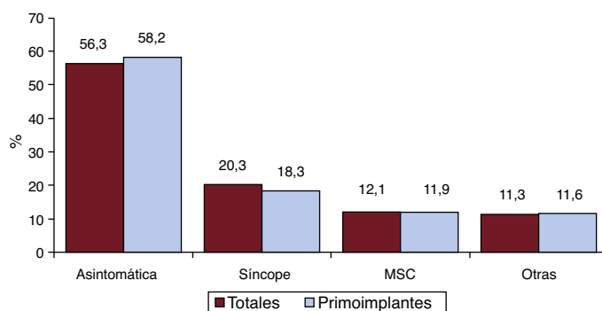
Figura 8. Forma de presentación clínica de la arritmia de los pacientes del registro (total y primoinplantes). MSC: muerte súbita cardíaca.
